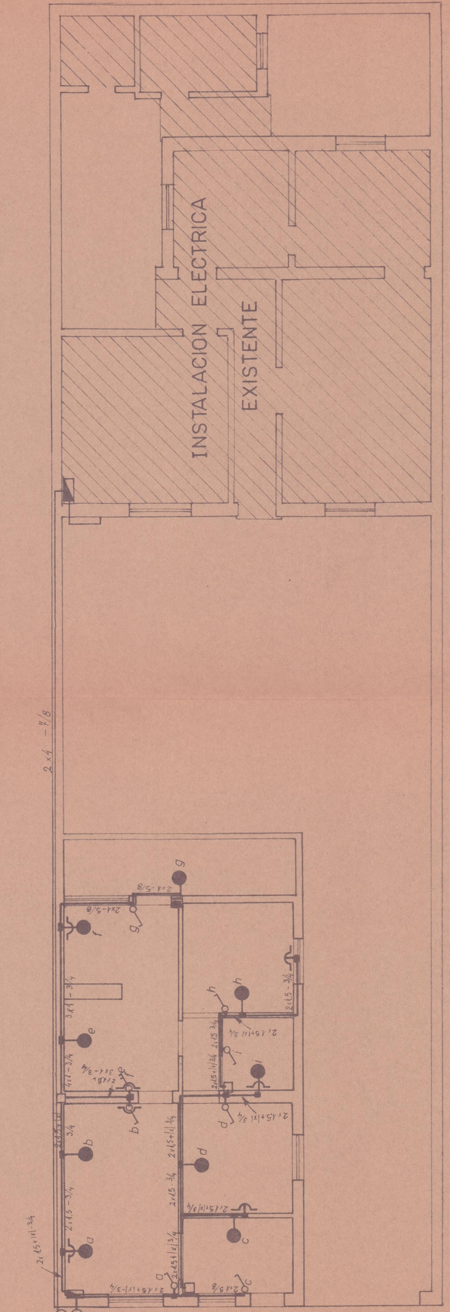
INSTALACION ELECTRICA
